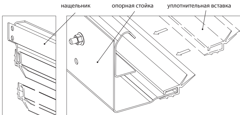
Рис. 7.1. Установка уплотнительной вставки
