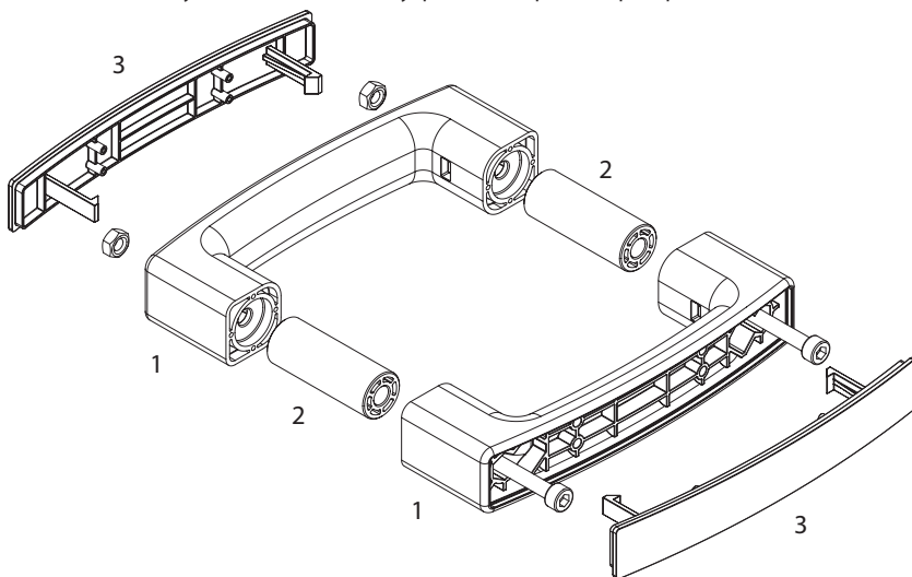
Рис. 39 Комплект ручки HGI006
