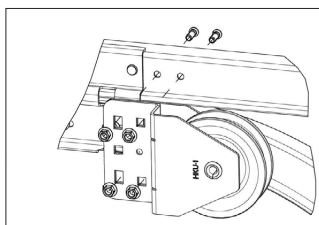
Рис. 43. Крепление блока НКU001 к горизонтальной направляющей
